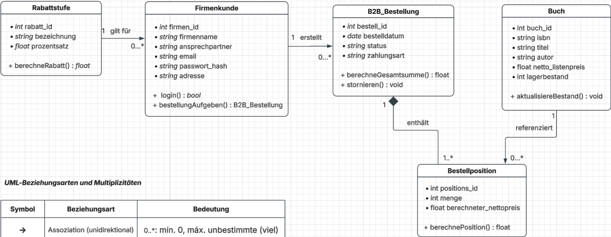
Klassendiagramm BookFly B2B
